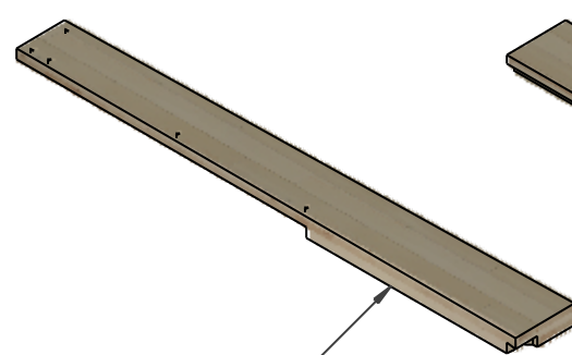
VS-7_CLT 1720x200x60 1x
