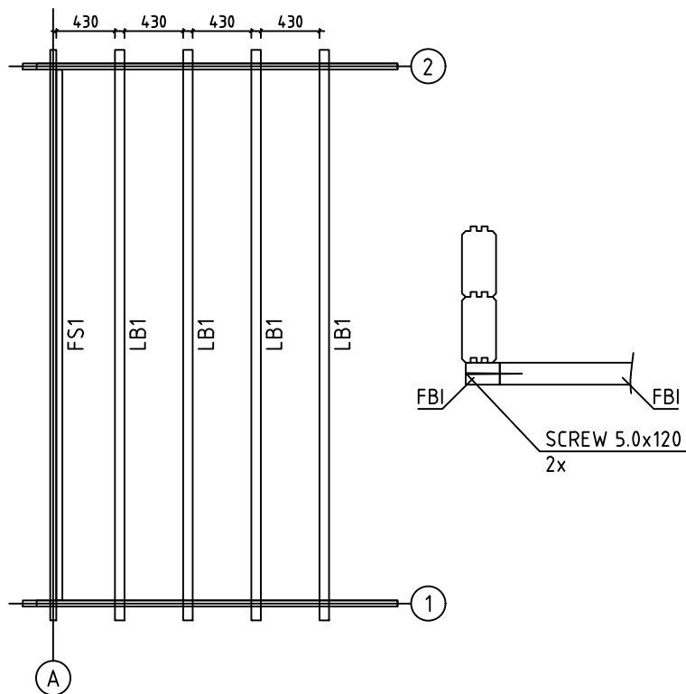
LOFT FLOOR BEAM- SCHLAFBODENBALKEN- SLAAPVLOERBALKEN
