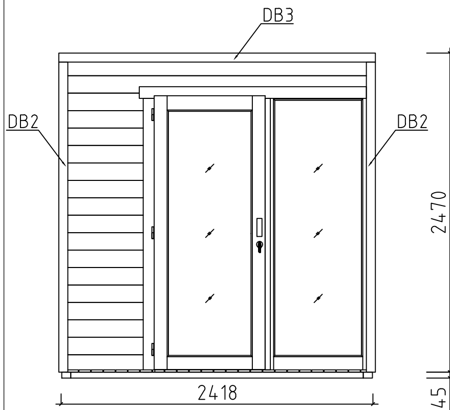
VORDERANSICHT- FRONT VIEW
