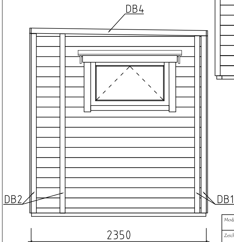
SEITENANSICHT (RECHTS) - SIDE VIEW (RIGHT)
