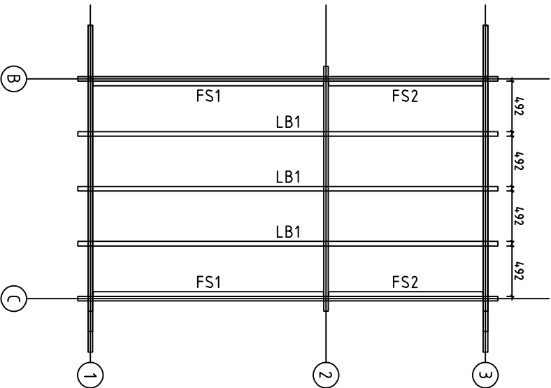
LOFT FLOOR BEAM- SCHLAFBODENBALKEN- SLAAPVLOERBALKEN
